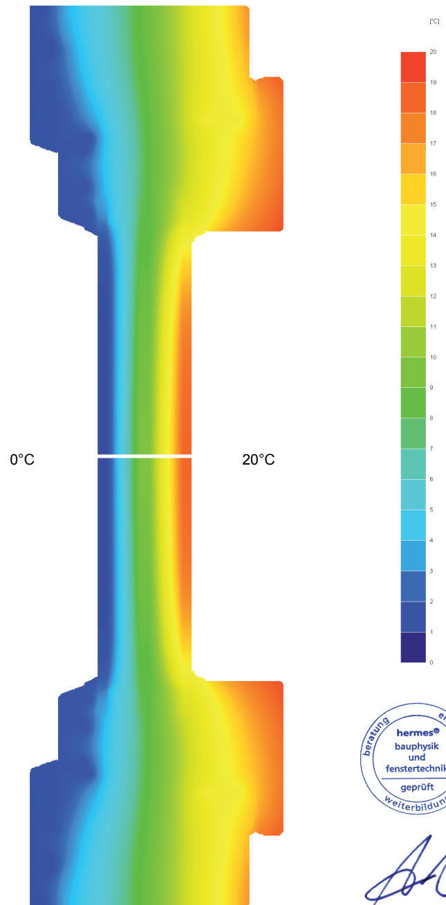
Temperaturfeld, farbig
