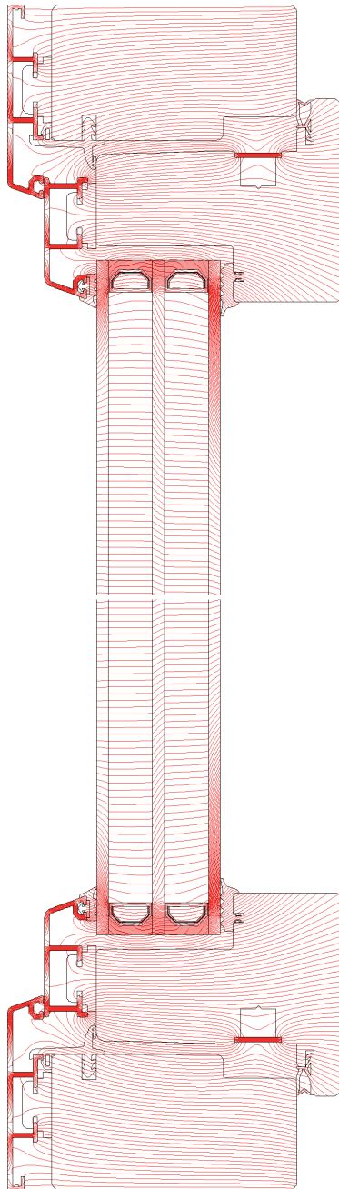
Verlauf der Wärmeströme
